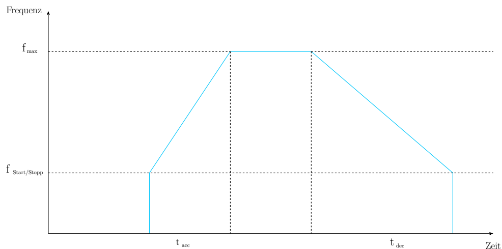
Abbildung 13.3.: Trapezförmiges Geschwindigkeitsprofil [Dr.20]
